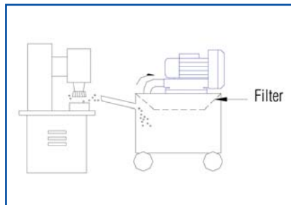
Aspiración industrial polvo Sucking Industrial Dust
